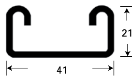
CH104 Weight 1.8 Kg/m
